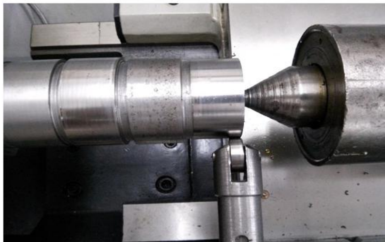
Рисунок 3 – Процесс работы роликового обкатника
