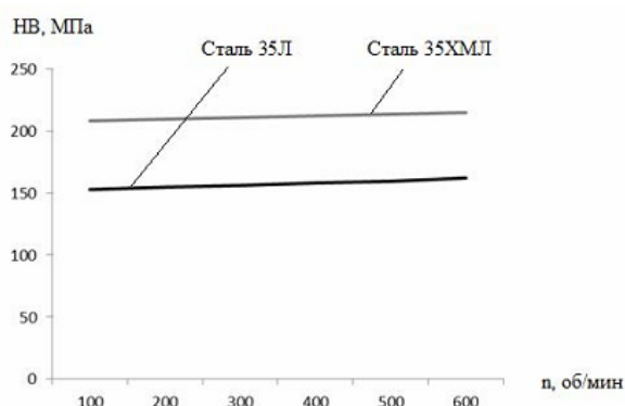
Рисунок 4 – Графики зависимости твердости поверхности HB = f(n) для сталей 35Л и 35ХМЛ при усилии обработки роликом P = 400 Н
